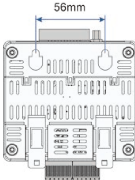
Abbildung 5-1 Befestigungsöffnungen
