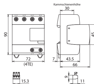
Maßbild
