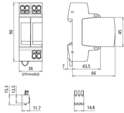
Maßbild DG MP TN 275 FM
