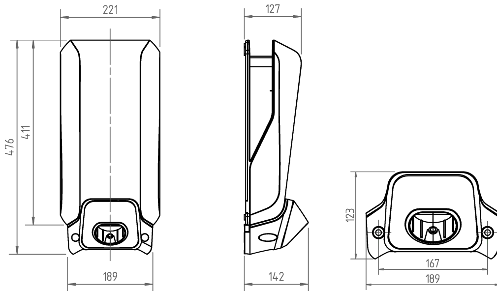
Abmessungen in Millimeter
