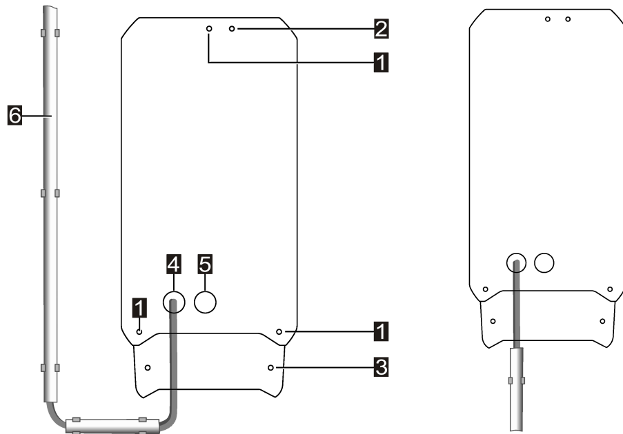
Abb. 8-3: Beispiel: Befestigungspunkte und Aufputz-Kabelverlegung
