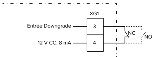
Fig. 17 : Schéma de principe : raccordement d'un contact électrique externe (réglage par défaut : NO)
