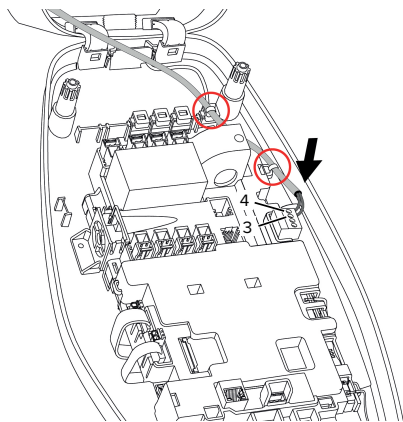
Kuva 16: Downgrade-tulon liitäntä
