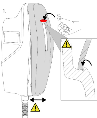
Kuva 21: Front Coverin kiinnitys – 1
