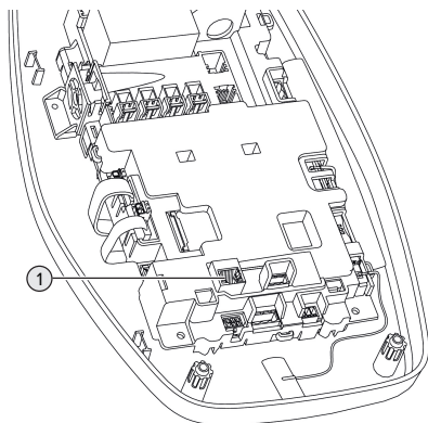
Fig. 14 : Prise Ethernet
