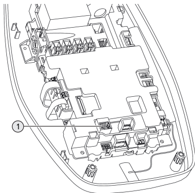
Fig. 14: Ethernet-anslutning
