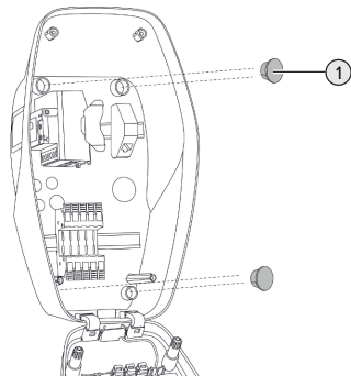
Obr. 9: Uzavírací zátky (příklad)
