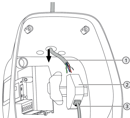
Fig. 15: Conexión del cable de datos (ejemplo)
