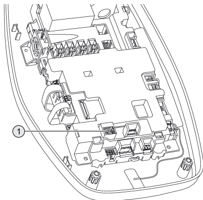
14. Ábra: Ethernet csatlakozás
