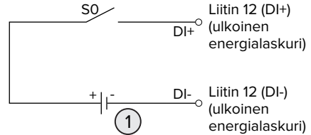
Kuva 18: Ohjaus kytkentäreleellä ja ylimääräisellä jännitesyötöllä (toimitustilassa)
