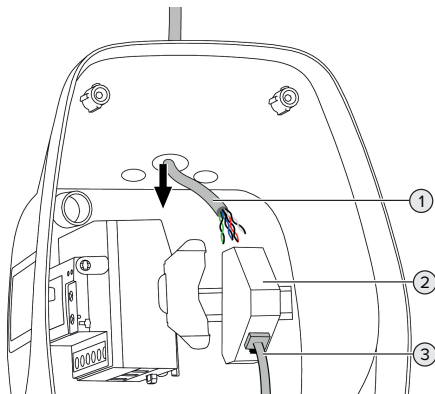
Ilustr. 15: Podłączenie przewodu danych (przykład)
