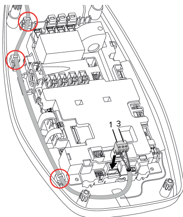
Fig. 11: Anslutning arbetsströmutlösare
