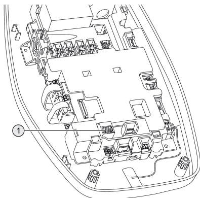
Ilustr. 14: Przyłącze Ethernet
