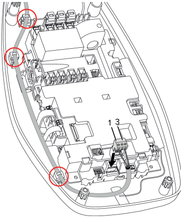
Fig. 11 : Raccordement du limiteur de courant de travail
