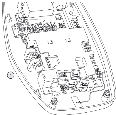
Afb. 14: Ethernet aansluiting
