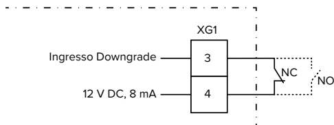
Fig. 17: Diagramma unifilare: collegamento di un contatto di commutazione esterno (impostazione di default: NO)
