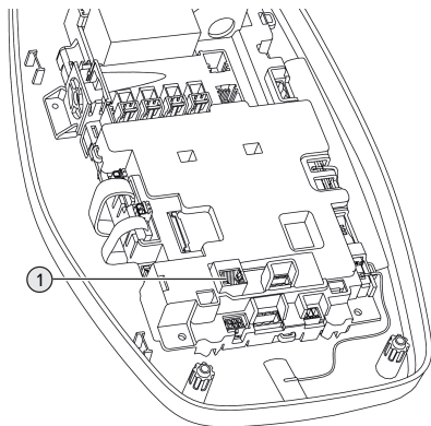
Fig. 14: Ethernet-tilslutning
