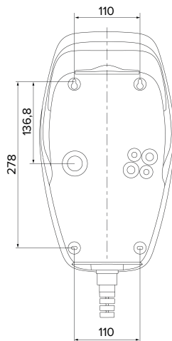
Kuva 7: Porausmitat [mm]
