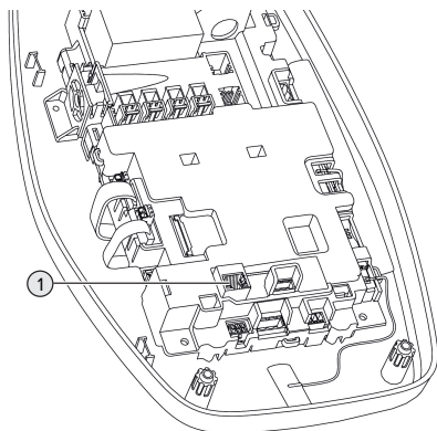
Obr. 14: Přípojka Ethernetu
