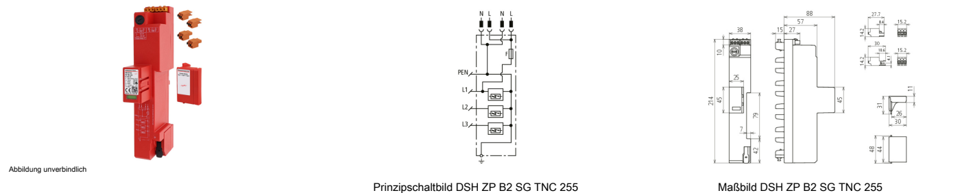
Abbildung unverbindlich Prinzipschaltbild DSH ZP B2 SG TNC 255 Maßbild DSH ZP B2 SG TNC 255 Kombi-Ableiter für TN-C-Systeme zum Einsatz im Hauptstromversorgungssystem (3+0-Schaltung) bei Wohngebäuden ohne äußeren Blitzschutz (auch mit Freileitungseinspeisung) inkl. überstromgeschützter 230 V Spannungsversorgung für RfZ / APZ nach VDE-AR-N 4100.
