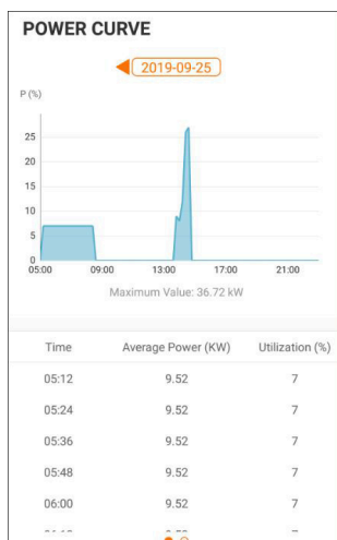
figure 7-10 Leistungsverlauf
