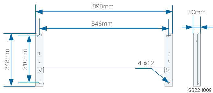
figure 4-1 Abmessungen des Befestigungswinkels
