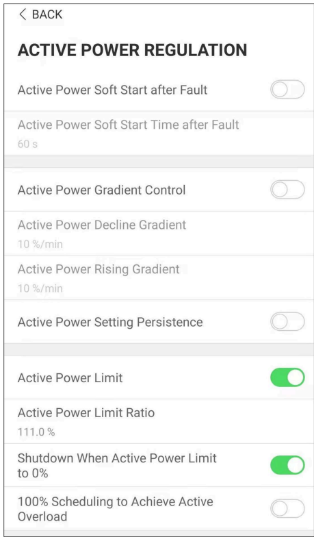
figure 7-17 Wirkleistungsregelung
