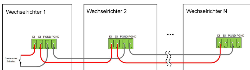
figure 5-11 Reihenschaltung
