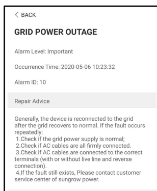
figure 7-9 Detaillierte Informationen einer Störungsmeldung
