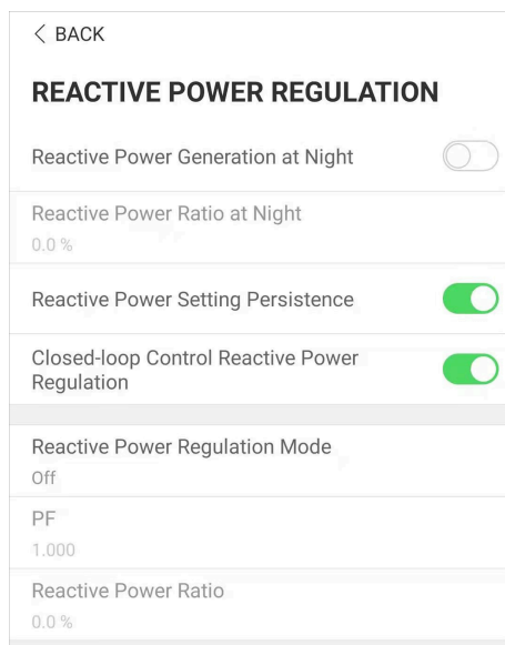
figure 7-18 Blindleistungsregelung
