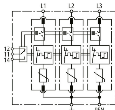
Prinzip Schaltbild DG M TNC ACI 275 FM
