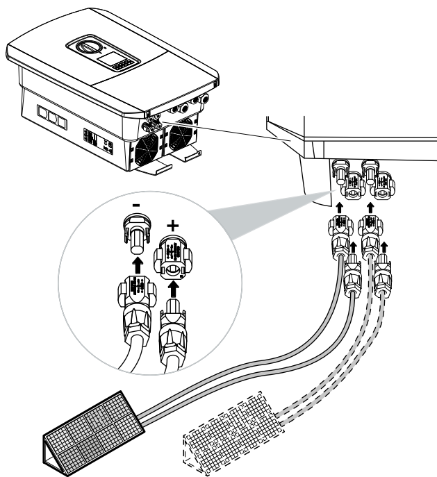
Abb. 35: Übersicht DC-Anschlüsse
