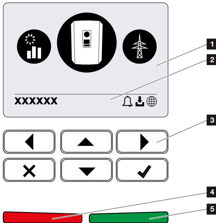
Abb. 12: Bedienfeld
