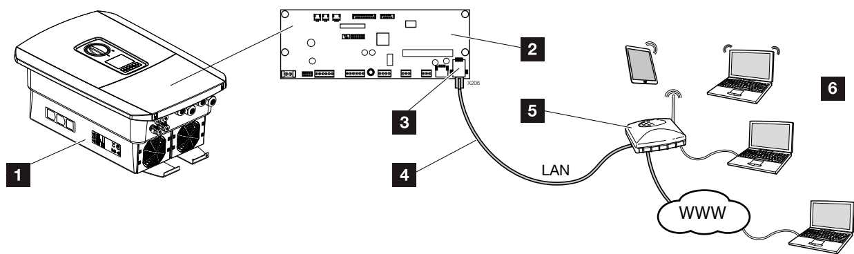
Abb. 31: Anschluss Kommunikation
