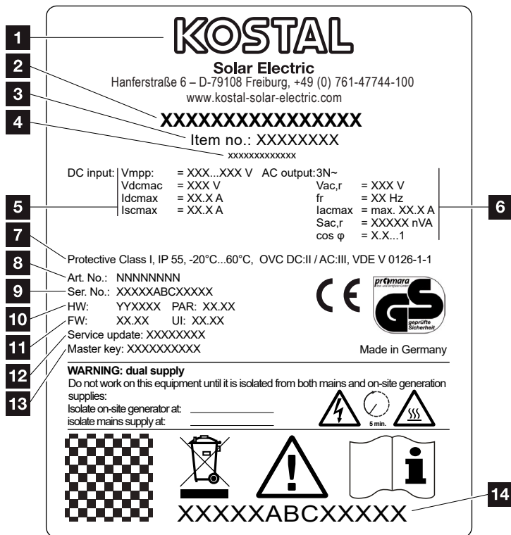
Abb. 68: Typenschild
