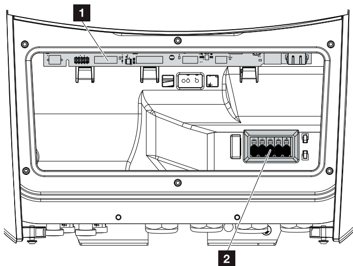
Abb. 11: Wechselrichter (Innenansicht)
