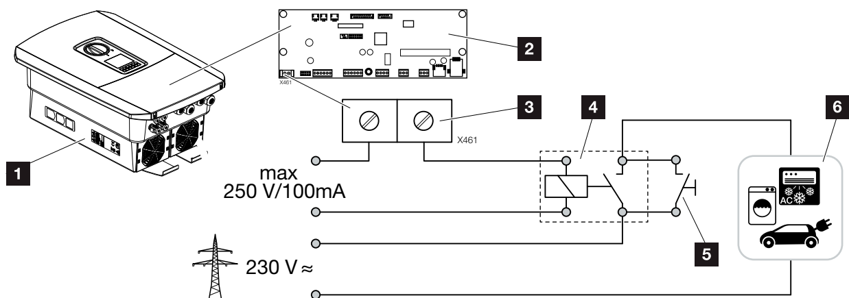
Abb. 30: Anschluss Eigenverbraucher
