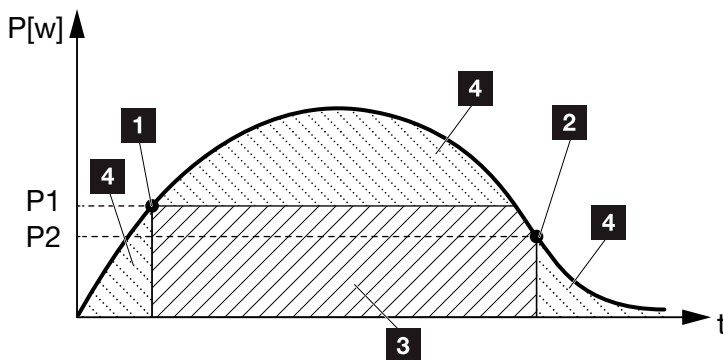
Abb. 58: Kurve Eigenverbrauch (Funktion 2)
