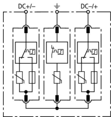
Prinzipialschaltbild DG M YPV SCI 1200
