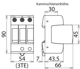
Maßbild DG M YPV SCI 1200
