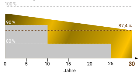
Modulleistung
