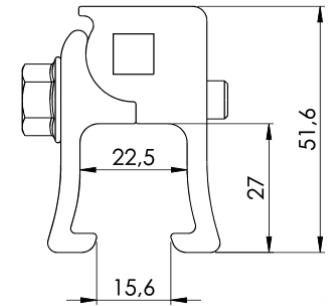
Falzklemme 2.1 K15 TPF
