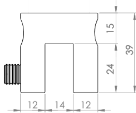
Winkelstehfalzklemme 2.1 TPF
