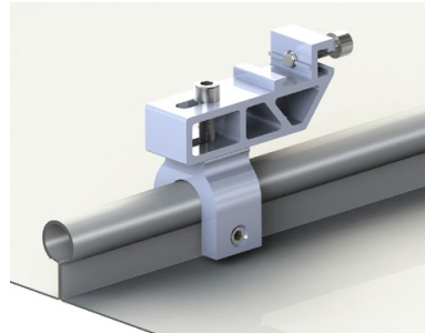
Rundfalz
