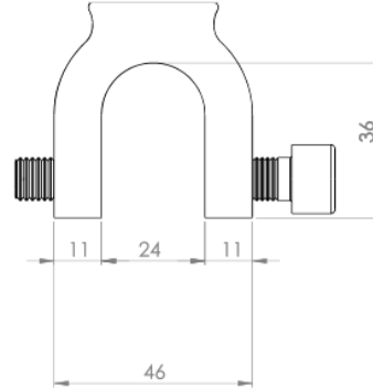
Rundfalzklemme 2.1 TPF
