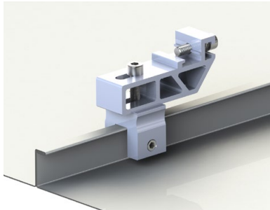
Winkelstehfalz
