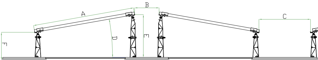
Reihenabstände SSL
