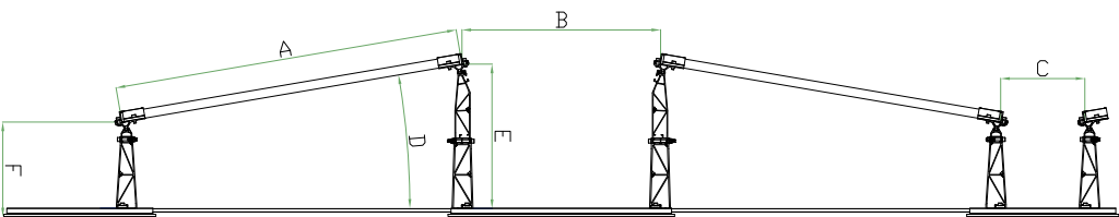
Reihenabstände SLS
