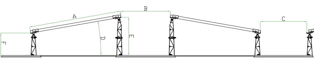
Reihenabstände SLL
