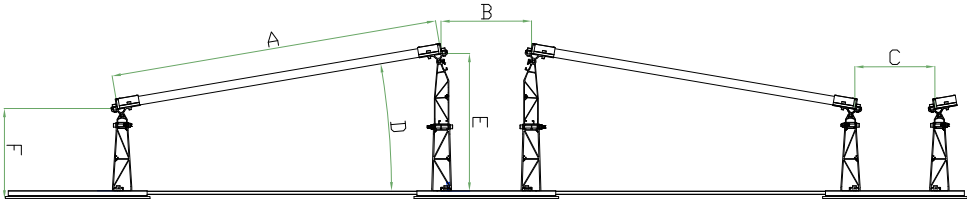
Reihenabstände SSS
