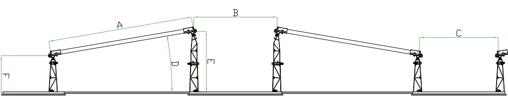
Reihenabstände SLL
