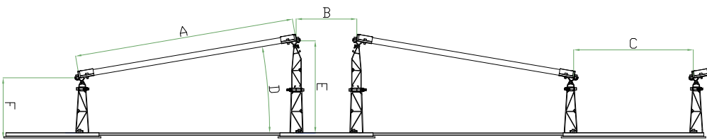
Reihenabstände SSL
