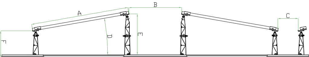
Reihenabstände SLS
