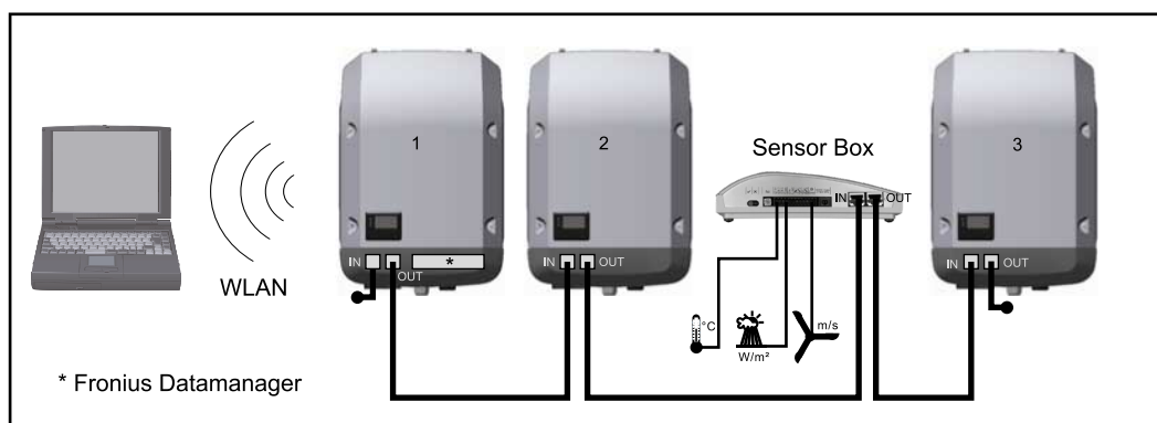
Datatenetwerk met 3 inverters en een Fronius Sensor Box: - Inverter 1 met Fronius Datamanager - Inverter 2 en 3 zonder Fronius Datamanager!
