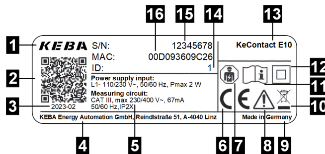
Abb. 4-4: Beispiel Typenschild
