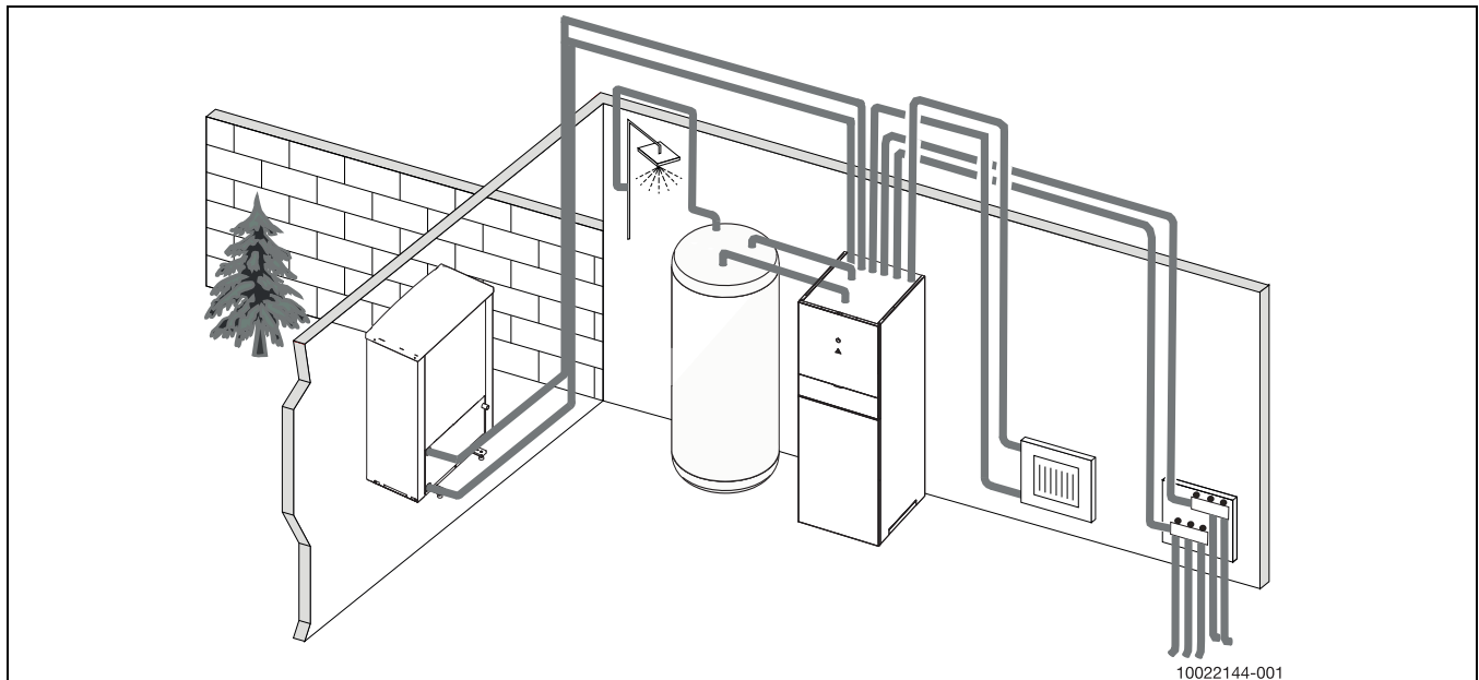
Bild 3 Wärmepumpe Compress 7001i AW, Inneneinheit AWMB mit integriertem Pufferspeicher und elektrischem Zuheizter, externer Warmwasserspeicher
