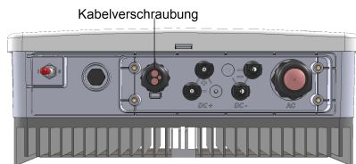
Abbildung 12: Kabelverschraubung Kommunikationsanschlüsse
