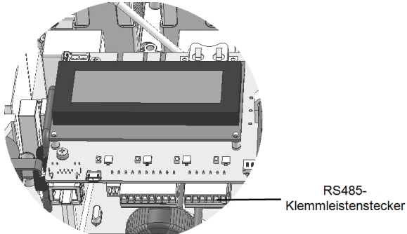
Abbildung 18: Die RS485-Klemmleiste
