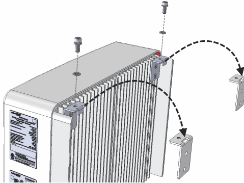
Abbildung 24: Montagehalterungen
