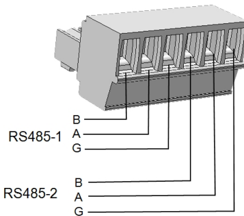
Abbildung 19: RS485-Klemmleistenstecker
