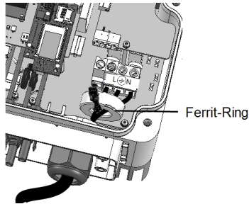
Abbildung 8: AC-Anschluss
