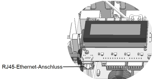
Abbildung 17: Die RJ45-Ethernet-Verbindung
