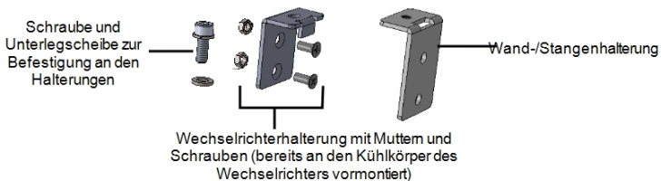
Abbildung 4: Montagehalterungen und Schrauben
