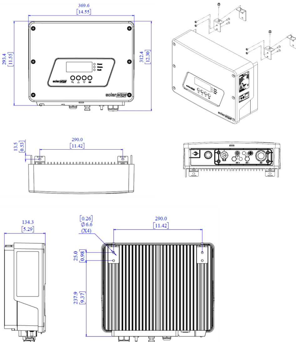
Abbildung 22: HD-Wave-Wechselrichter-Abmessungen
